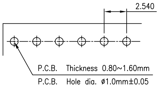
PCB LAOUT
