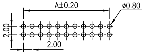
P.C.B LAYOUT
