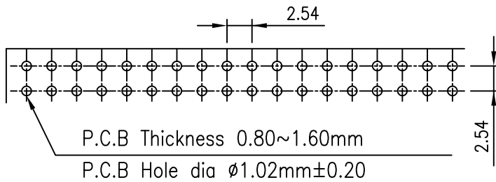
P.C.B. LAYOUT
