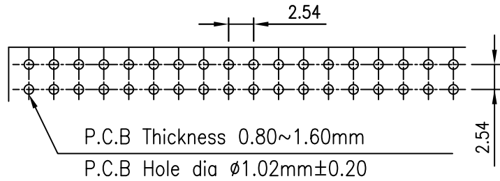
P.C.B. LAYOUT
